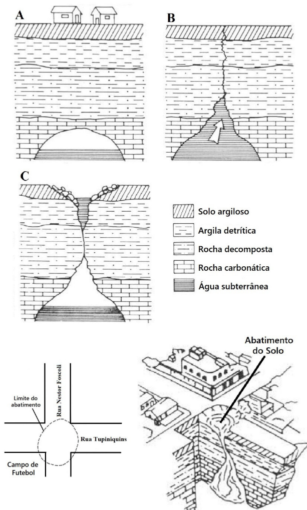
Figura 6 – Fases de evolução do abatimento do solo ocorrido em 4 de março de 1988, na cidade de Sete Lagoas/MG
