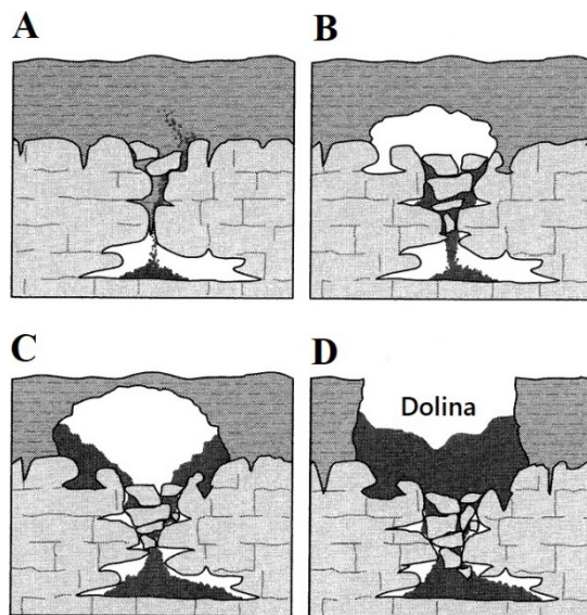
Figura 5 – Processo de formação de uma dolina de colapso
