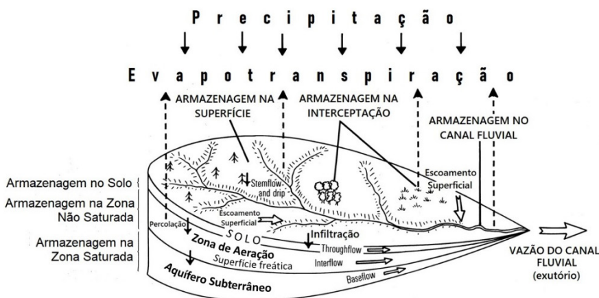
Figura 1 – Migração e armazenagem da água em uma bacia hidrográfica. Fonte: Summerfield (1991, p. 191, adaptado.).
