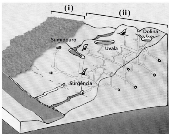
Figura 4 – A paisagem cárstica nem sempre revelada
